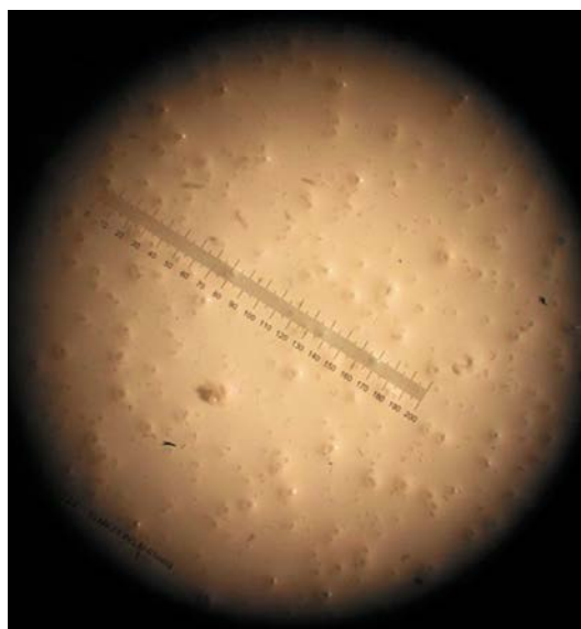
Gros plan du revêtement PU-PA, grossi 40 fois au microscope
