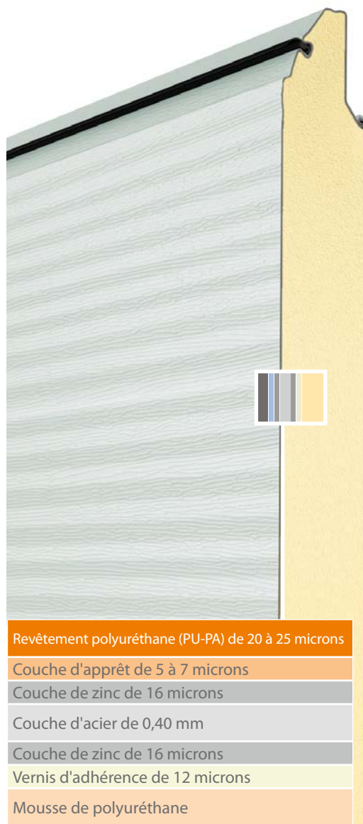
Composition de la tôle d'acier du panneau sandwich ALUTECH
