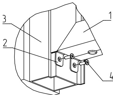
Рис. 21. Крепление фальш-панели к столбам калитки:
