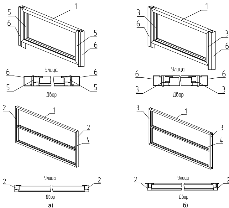
Рис. 1. Рама секции ограждения и горизонтальное сечение:
