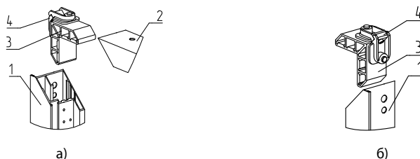
Рис. 2. Установка соединителей:
