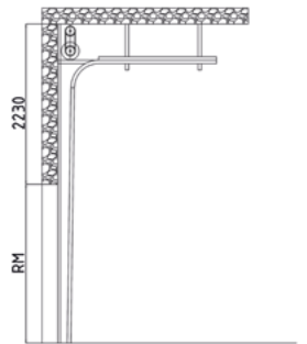
Высокий тип монтажа с верхним расположением вала
