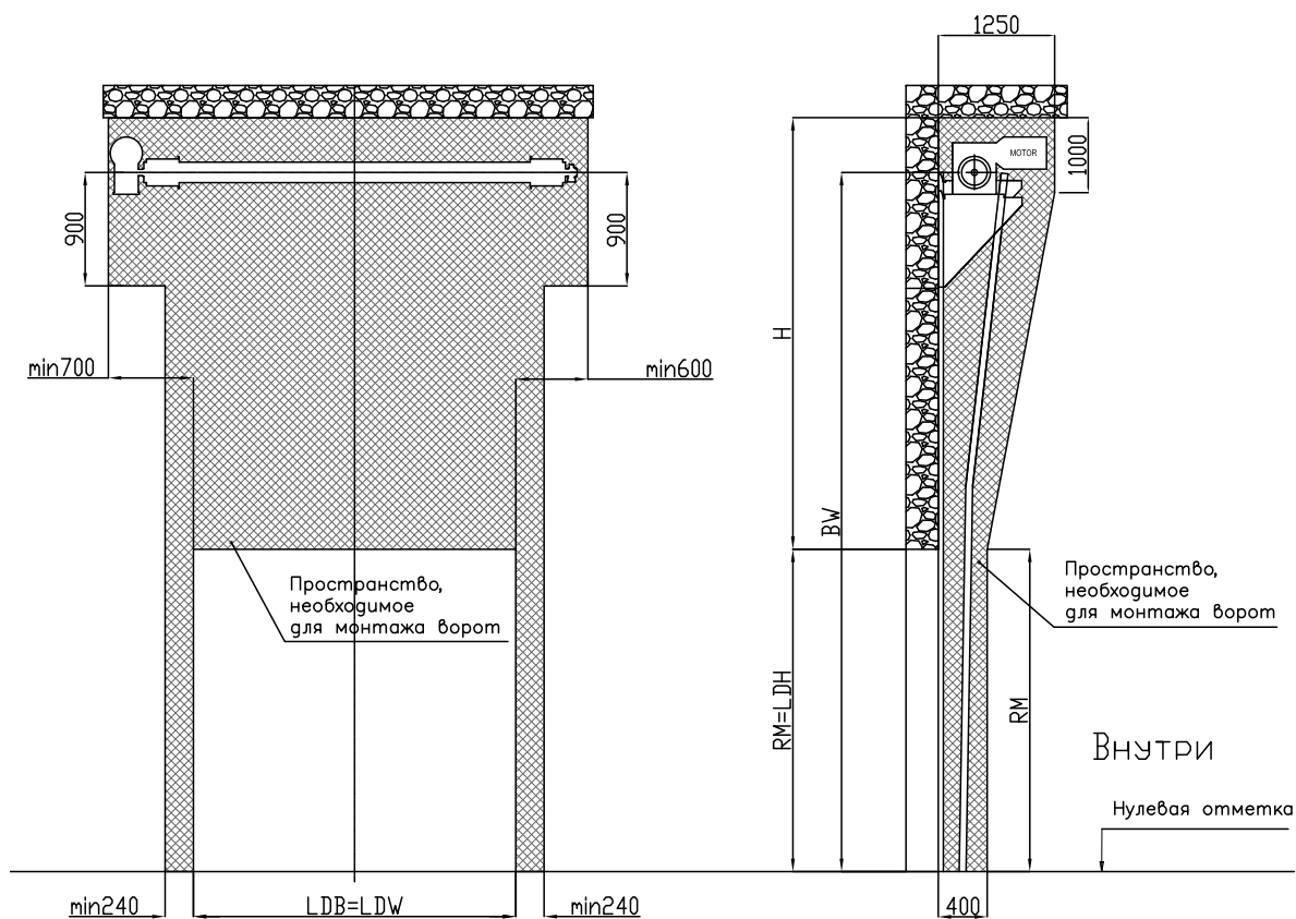
Тип балансировки см. табл. размерной сетки
