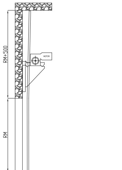
Вертикальный тип монтажа с нижним расположением вала
