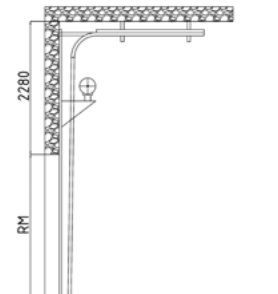
Высокий тип монтажа с нижним расположением вала
