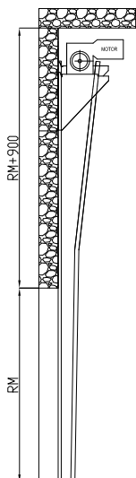
Вертикальный тип монтажа с верхним расположением вала
