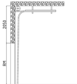
Высокий тип монтажа с верхним расположением вала
