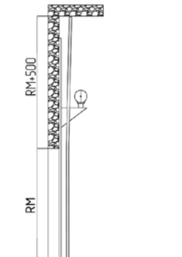
Вертикальный тип монтажа с нижним расположением вала
