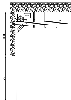
Высокий тип монтажа с верхним расположением вала
