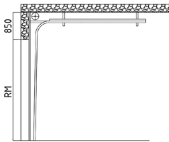
Стандартный тип монтажа
