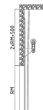
Вертикальный тип монтажа с нижним расположением вала
