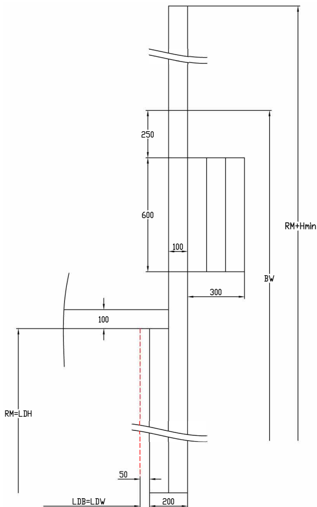
Одновальная система балансировки
