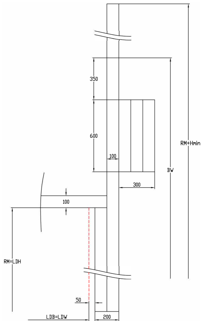
Двухвальная система балансировки
