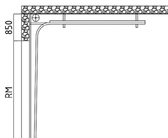
Стандартный тип монтажа
