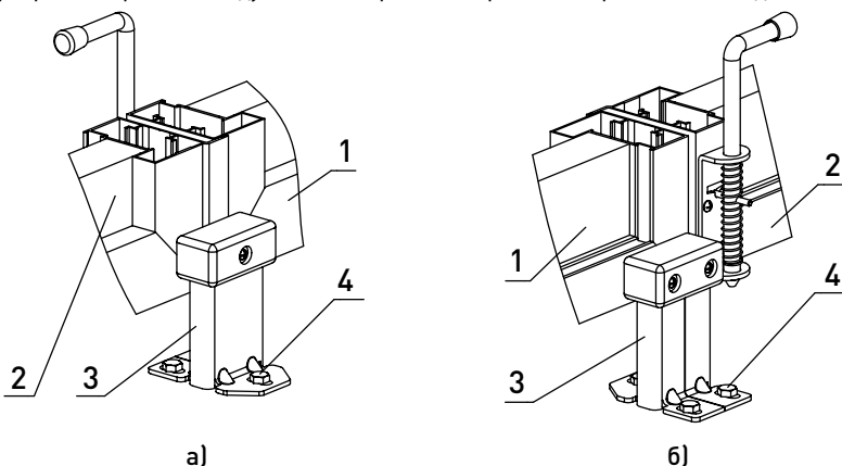
Рис. 60. Установка упора FLGU.400.0934 :
