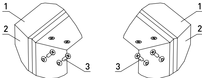
Рис. 49. Крепление перекладины к столбам ворот
