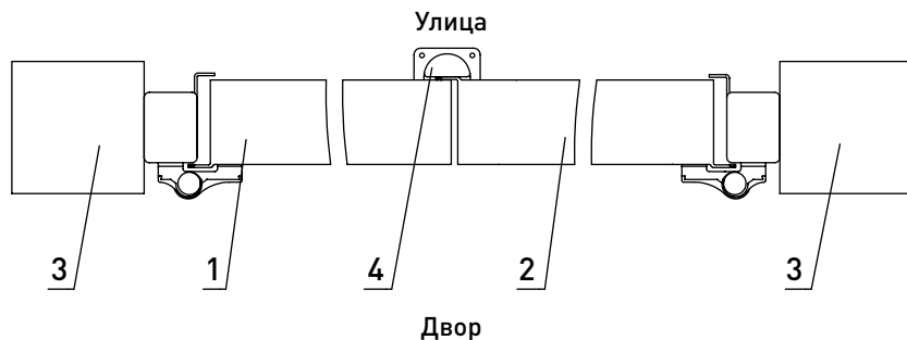
Рис. 53. Распашные ворота (встроенный тип монтажа, вид открывания внутрь)
