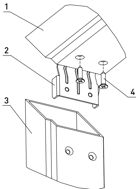
Рис. 48. Крепление соединителя углового FLGU.400.0944
