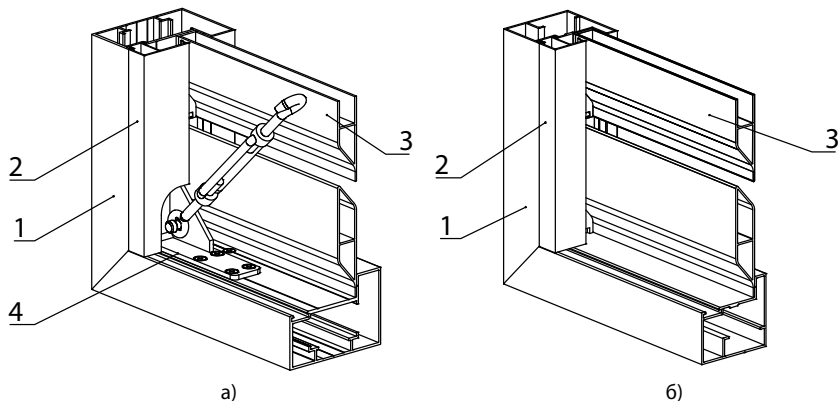
Рис. 39. Установка штапиков FLGU.400.0302, FLGU.400.0304 в раму с заполнением «жалюзи»:
