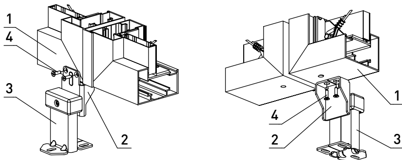
Рис. 61. Установка упора FLGU. 400. 0935
