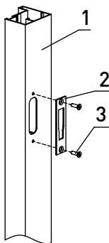
Рис. 51. Установка ответной планки комплекта запирания
