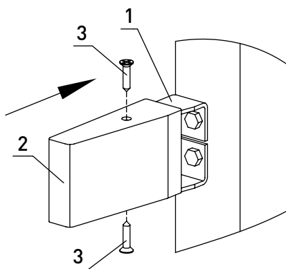
Рис.56. Установка крышки FLGU.400.0722
