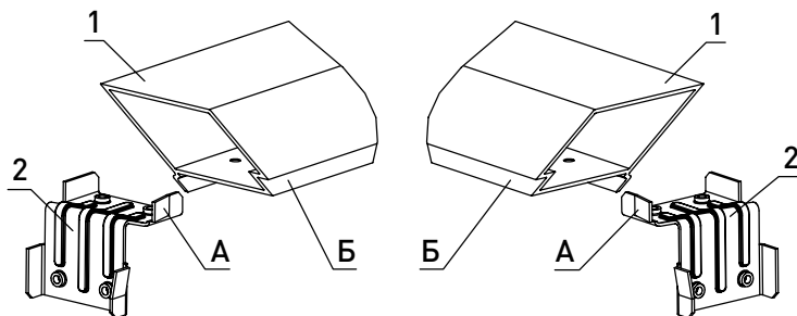
Рис. 47. Установка соединителей угловых FLGU.400.0944
