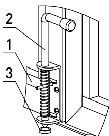
Рис. 64. Установка втулки FLGU.400.0915
