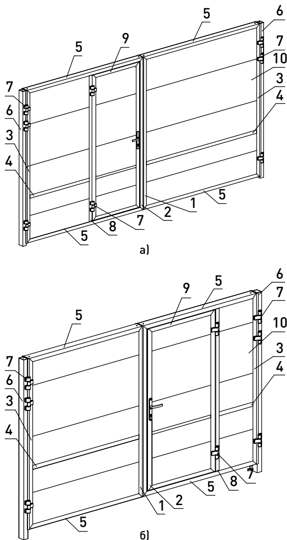
Рис. 69. Распашные ворота со встроенной калиткой (вид открывания внутрь):
