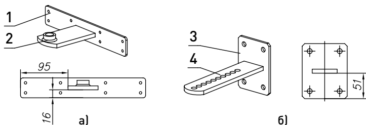
Рис. 65. Изготовление кронштейнов для установки электроприводов:
