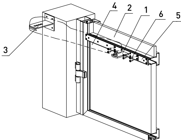
Рис. 67. Установка кронштейна для крепления электропривода
