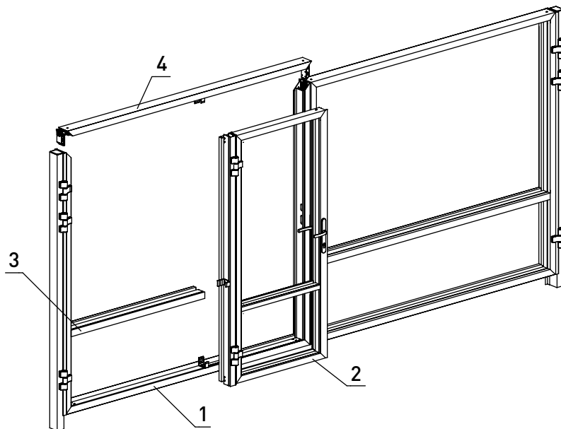
Рис. 71. Установка рамы калитки в створку распашных ворот
