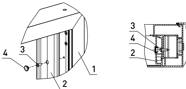
Рис. 72. Установка профиля притвора FLGU.400.0505
