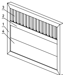
Рис. 40. Створка с комбинированным заполнением
