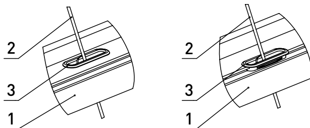
Рис. 45. Установка вставки:
