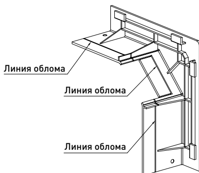
Рис. 21. Крышка FLGU.400.0717
