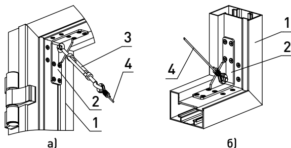
Рис. 442. Установка тросовой растяжки с талрепом:
