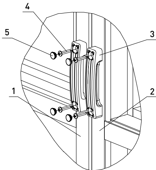
Рис. 58. Установка ручек
