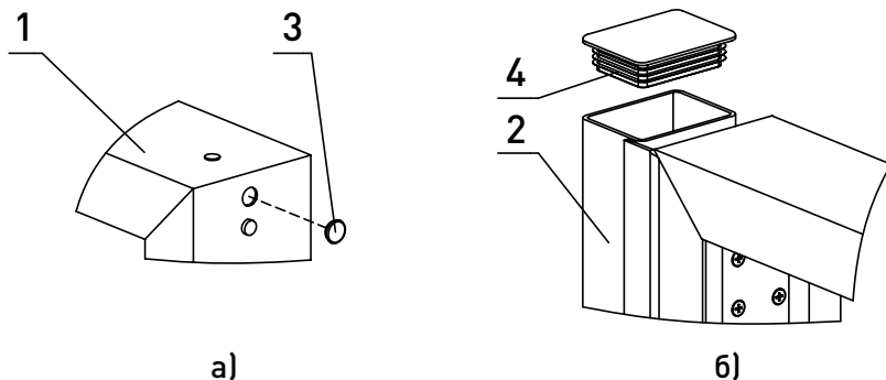
Рис. 43. Установка декоративных крышек:
