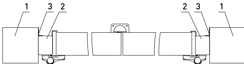
Рис. 68. Установка профиля притвора АУРС.120.0201
