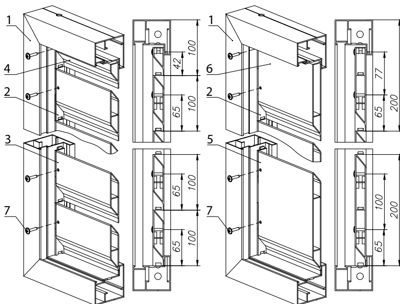
Рис. 37. Заполнение алюминиевым профилем «жалюзи»:
