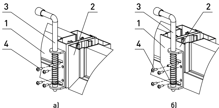
Рис. 59. Установка засова:
