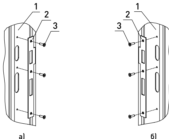
Рис. 73. Установка ответной пластины:
