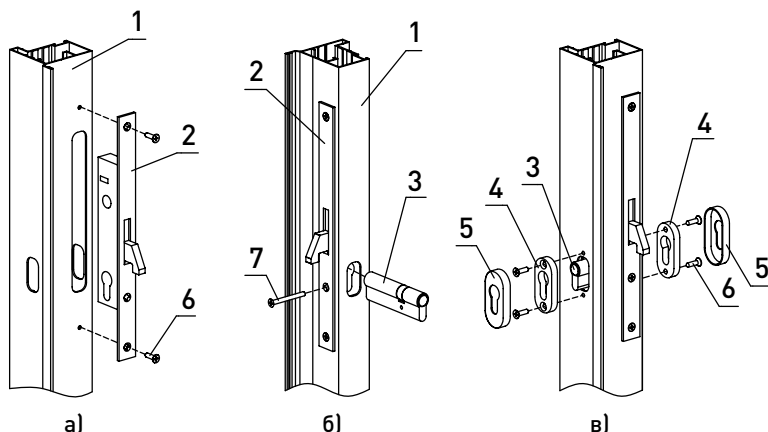
Рис. 50. Установка комплекта запирания
