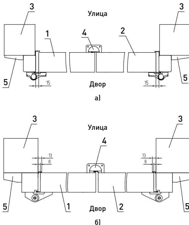
Рис. 54. Распашные ворота (накладной тип монтажа, вид открывания внутрь):
