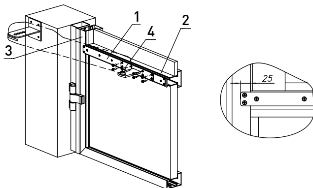
Рис. 66. Установка пластин FLGU.400.0952 (FLGU.400.0953)
