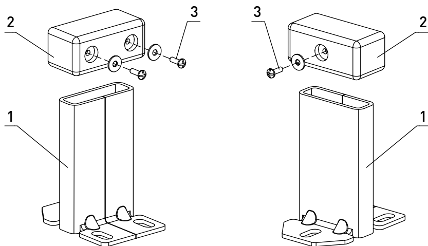
Рис. 63. Сборка упора FLGU.400.0934
