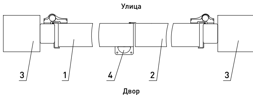
Рис. 52. Распашные ворота (встроенный тип монтажа, вид открывания наружу)
