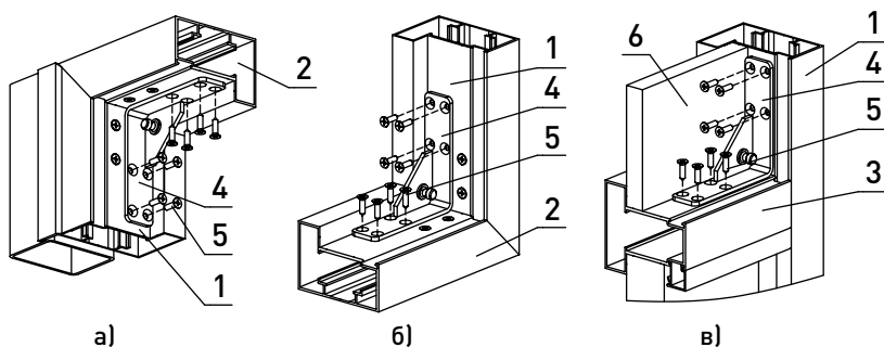
Рис. 41. Установка кронштейна FLGU.400.0906 :
