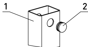
Рис. 57. Установка декоративной заглушки
