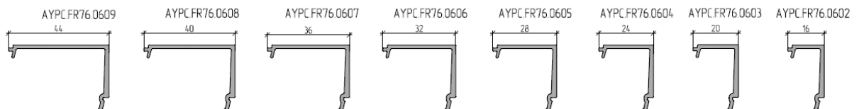
Оригинальные профили штапиков FR76
