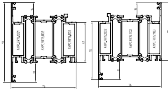
Профили створки
