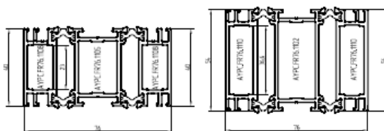
Профили уширителя
