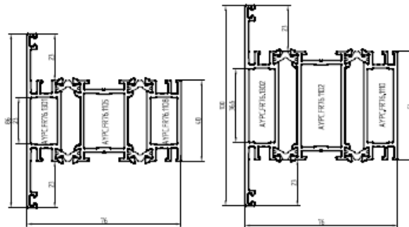
Профили импоста
