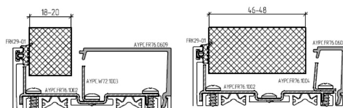
Оригинальные профили штапиков FR76
