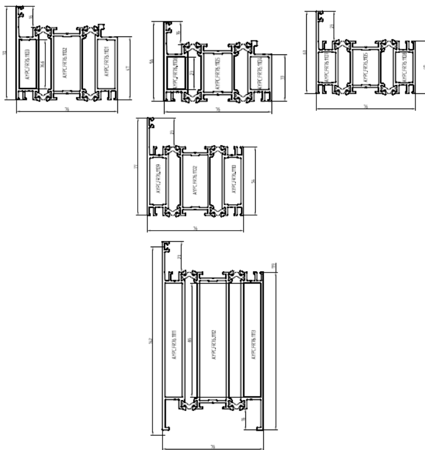
Профили рамы
