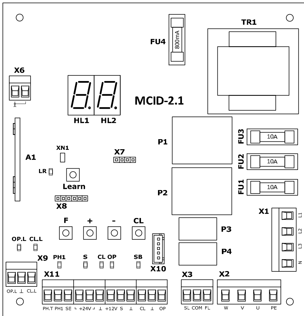
Рис. 1. Электронный модуль блока управления
