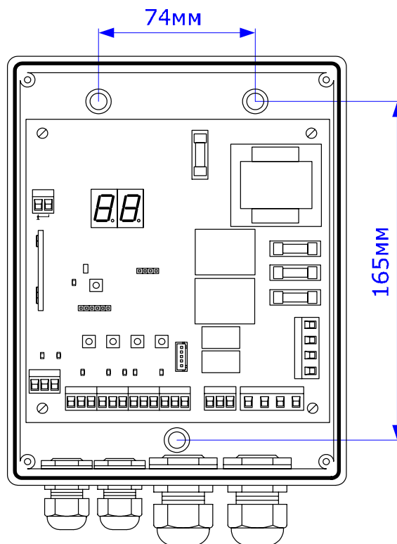
Рис. 2. Монтаж блока управления
